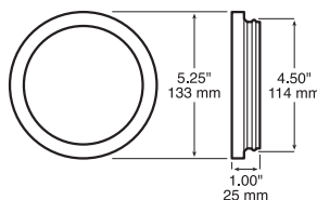
PM-B426-18 grommet
