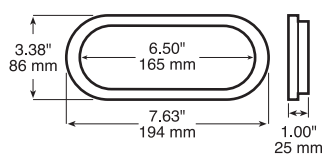
PM-B421-18 grommet
