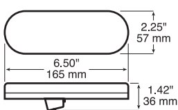
PM-1220R-10 light module
